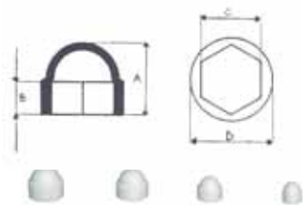
Tapón para tornillo
